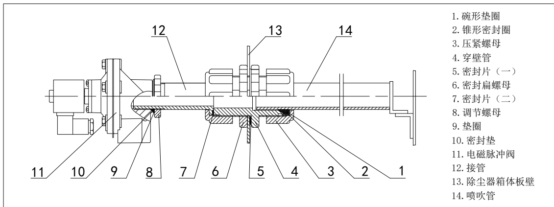
图26 FAP-A-3型安装图
