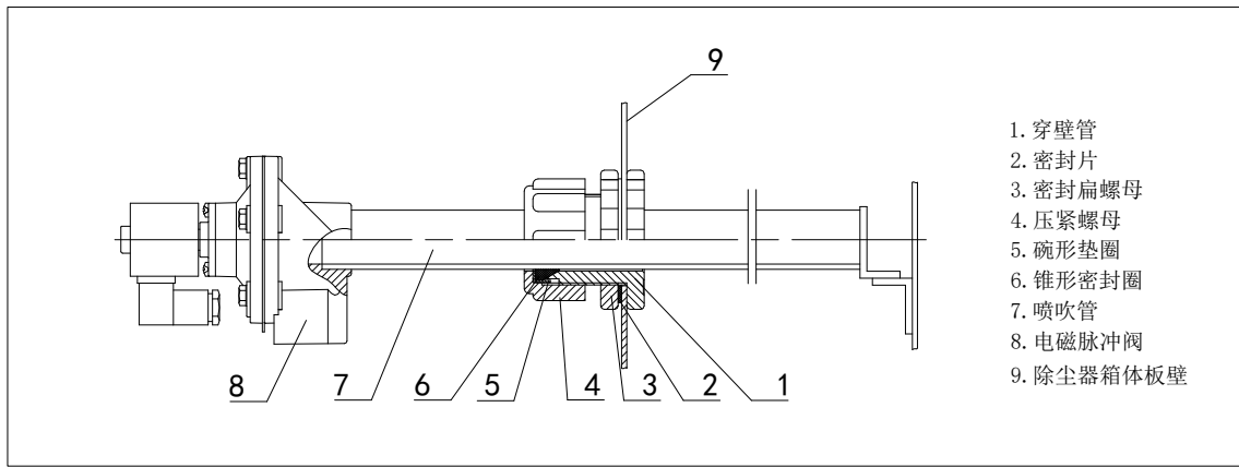
图24 FAP-A-1型安装图
