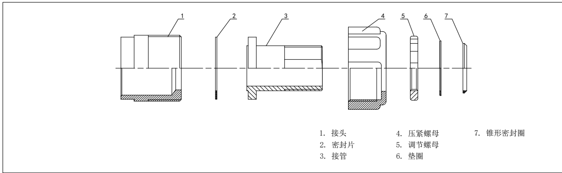
图6 FAP-C-1型结构图
