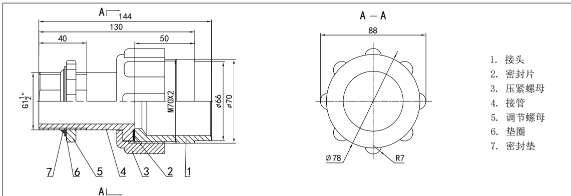
图23 FAP-C-1-40 外形尺寸图
